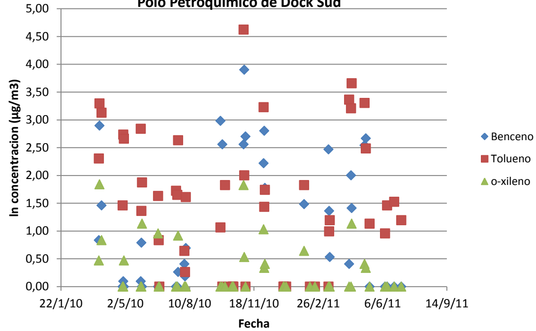
Concentraciones de benceno, tolueno y o-xileno (Marzo 2010 - Julio 2011) Polo Petroquímico de Dock Sud
